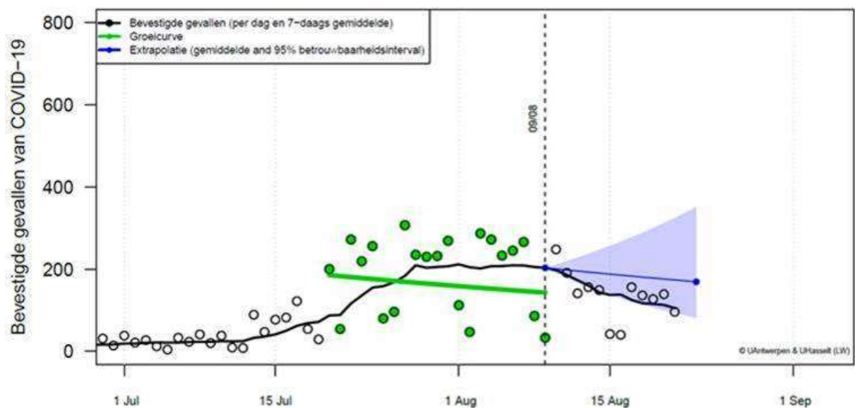
Grafiek 2: Groeimodel en voorspeld aantal bevestigde COVID-19-gevallen provincie Antwerpen op 09/08
