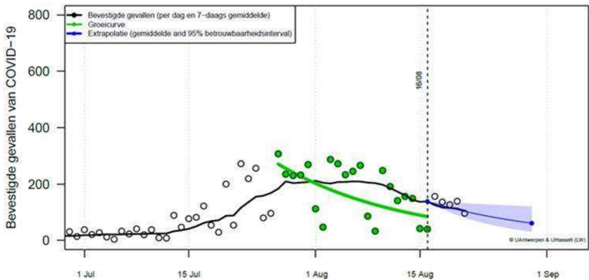
Grafiek 3: Groeimodel en voorspeld aantal bevestigde COVID-19-gevallen provincie Antwerpen op 16/08
