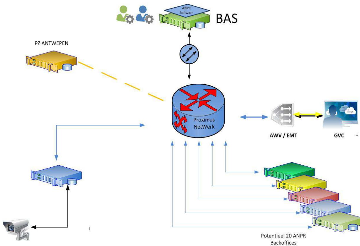
Figuur 14: Schematische voorstelling BAS.
