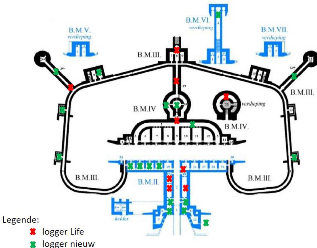
Figuur 10: Situering loggers in het fort van Duffel (vocht- en temperatuursmeting)
