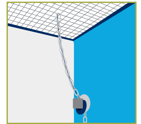
↑ 83 Goede vergrendeling van een kelderrooster.
