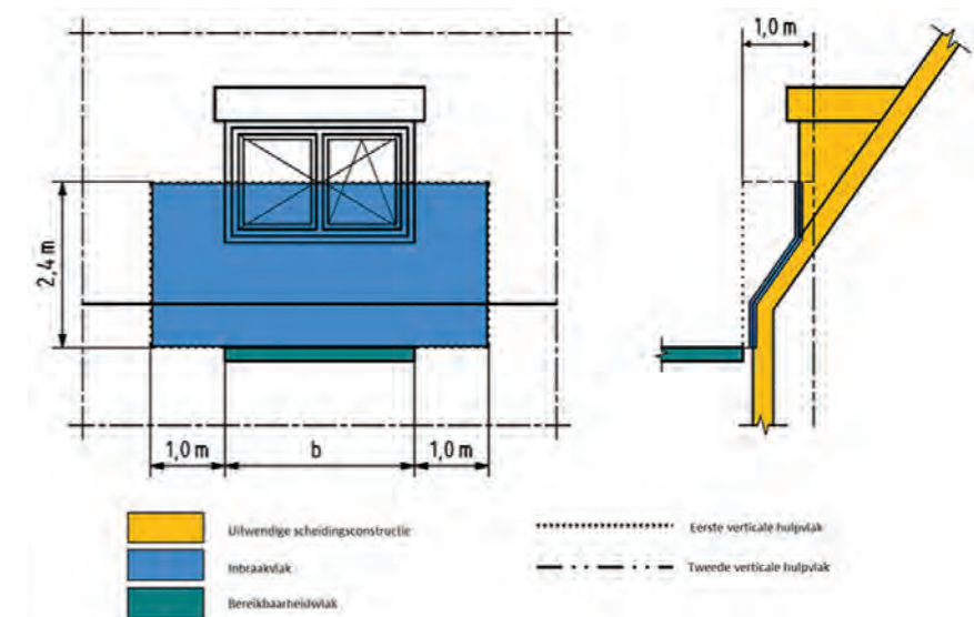
†3 Bereikbaarheidsvlakken van dak en gevel
