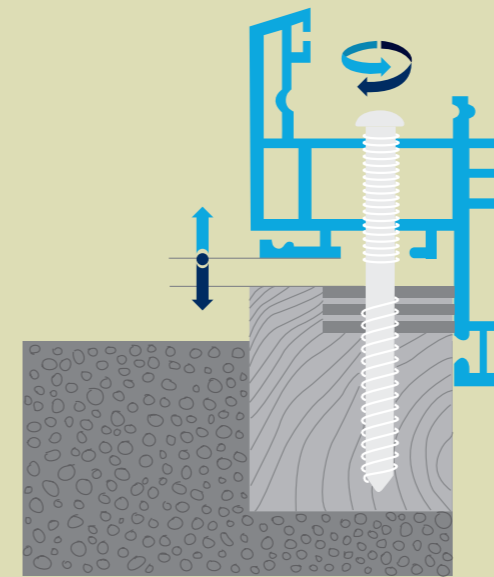
187 Bevestiging met schroef met dubbele draad.
