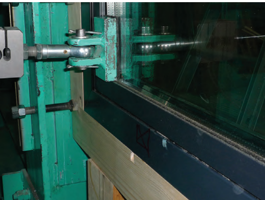
6 Statische proef.
