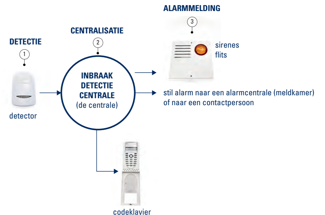
t89 De verschillende componenten van een alarmsysteem.
