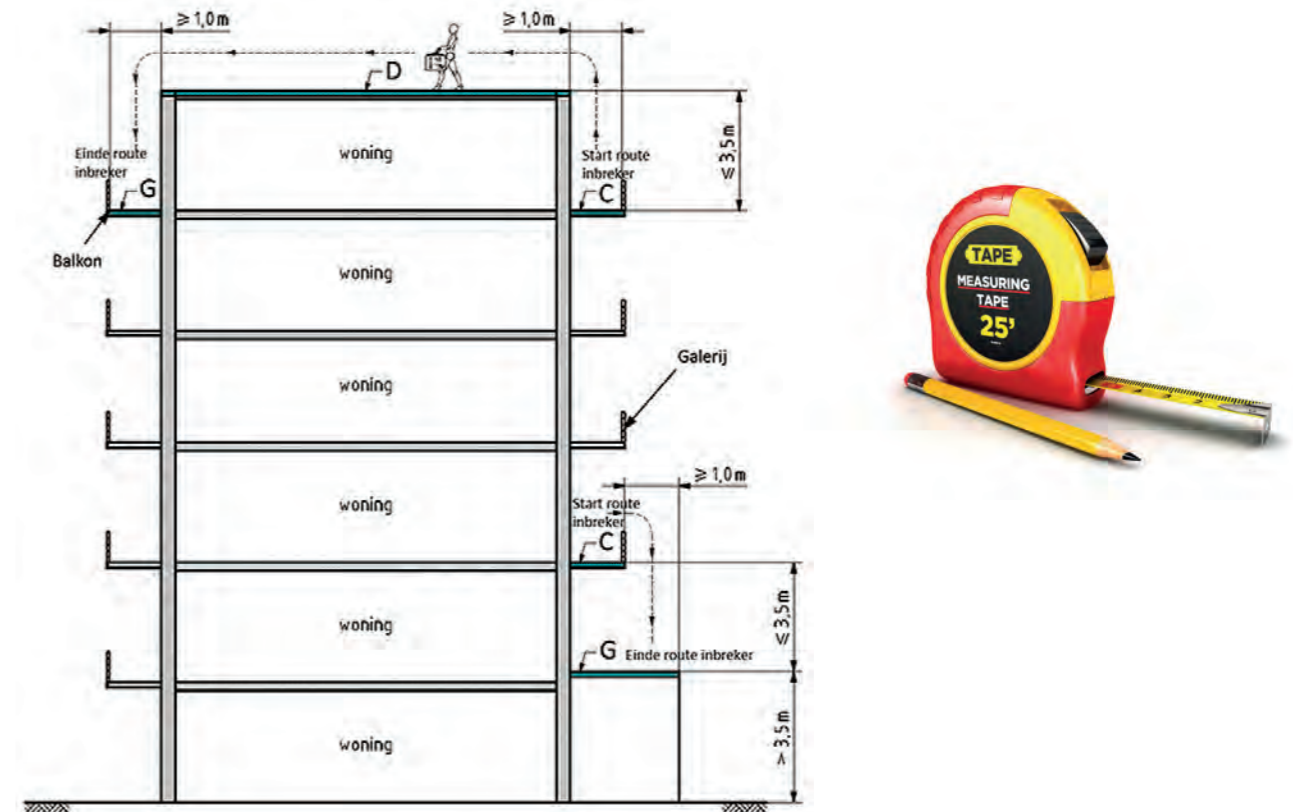
†2 Bereikbaarheidsvlakken van een appartementsgebouw
