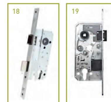
↑ 18 Buitenaanzicht van een standaard 1 puntscilinderslot met dag- en nachtschoot.
