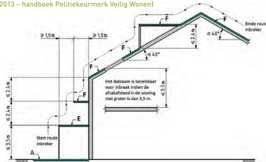
†1 Bereikbaarheidsvlakken van een woning met uitbouw.
